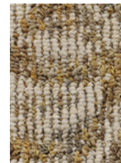
7831 Giotto
