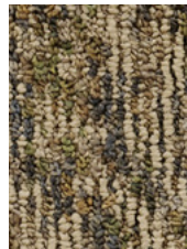
7836 Raphael
