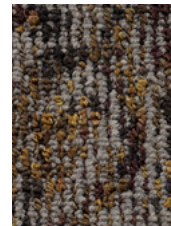
7978 Rubens
