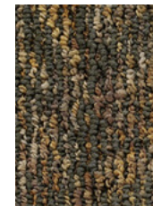
7689 Leonardo
