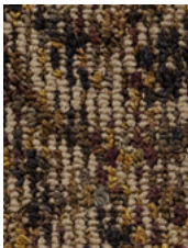
7858 Masolino
