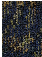
7596 Caravaggio
