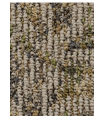
7848 Lippi
