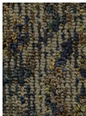
7668 Botticelli
