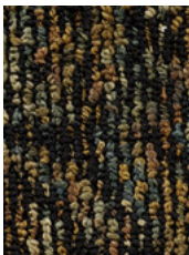
7988 Angelico
